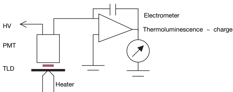
FIG. 3.8. TLD reader.
